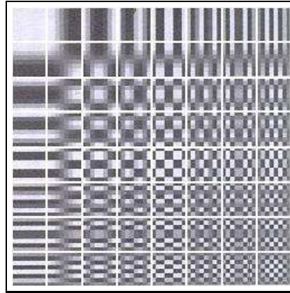
Figura 2.4: Padrão da base da DCT 8 \times 8 .
