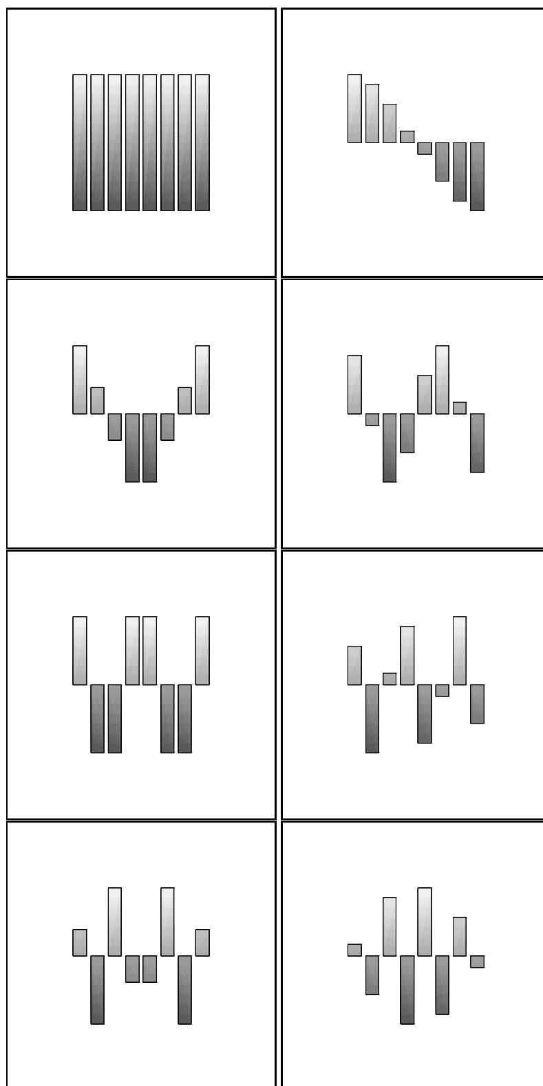
Figura 2.3: Conjunto de medidas para a base da DCT.
