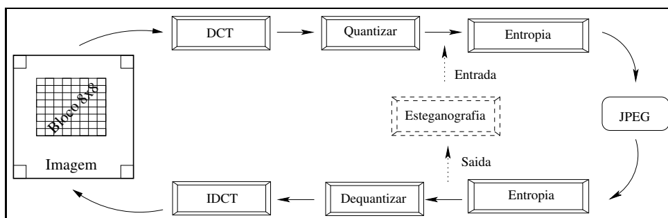
Figura 4.6: Esquema de esteganografia em JPEG.
