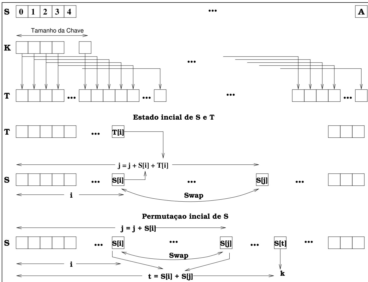
Figura 3.1: Esquema do RC4.
