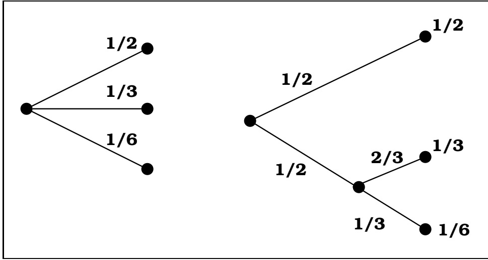
Figura 2.1: Decomposição de uma escolha de três possibilidades.
