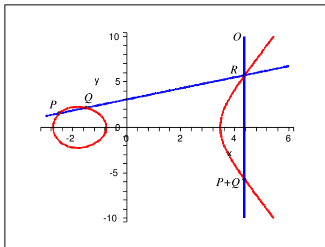
Figura 3.2: P + Q = -R .
