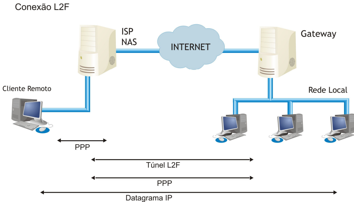
Figura 24 – Conexão L2F
