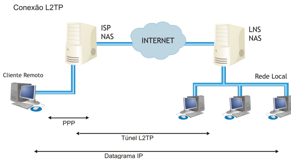
Figura 25 – Conexão L2TP
