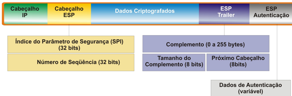
Figura 30 – Pacote ESP
