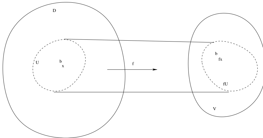
FIGURA 1. Continuidade de \mathbf{f}(\mathbf{x}) .
