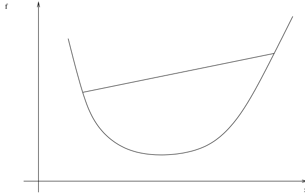
FIG. 8. Função convexa.
