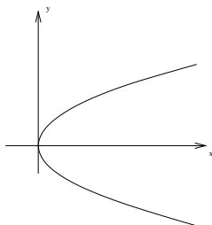
FIG. 11. Conjunto \{(x, y) \in \mathbb{R}^2 : x = y^2\} .
