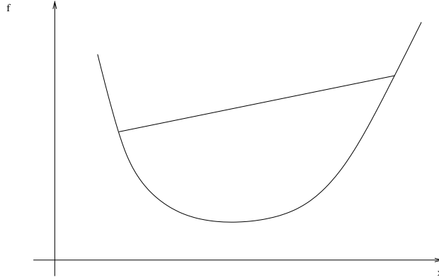
FIG. 8. Função convexa.
