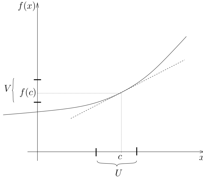
FIG. 9. Teorema da função inversa.
