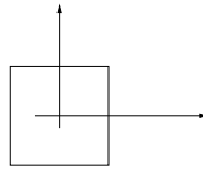
FIG. 2. Conjunto \{\mathbf{x} \in \mathbb{R}^2 : \|\mathbf{x}\|_\infty = 1\}
