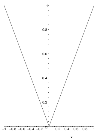
FIG. 2. Gráfico de f(x) = |x| , função contínua mas não diferenciável.
