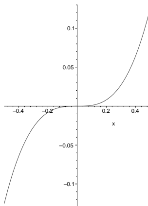
FIG. 3. Gráfico de f(x) = x^3 , que tem derivada zero em x = 0 , mas este não é ponto extremo.
