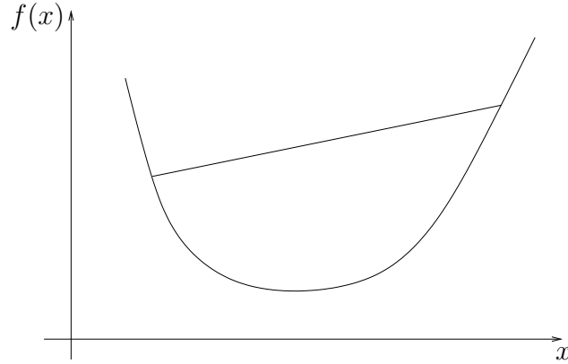
FIG. 8. Função convexa.
