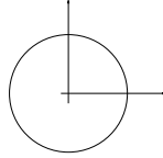
FIG. 1. Conjunto \{\mathbf{x} \in \mathbb{R}^2 : \|\mathbf{x}\| = 1\} .
